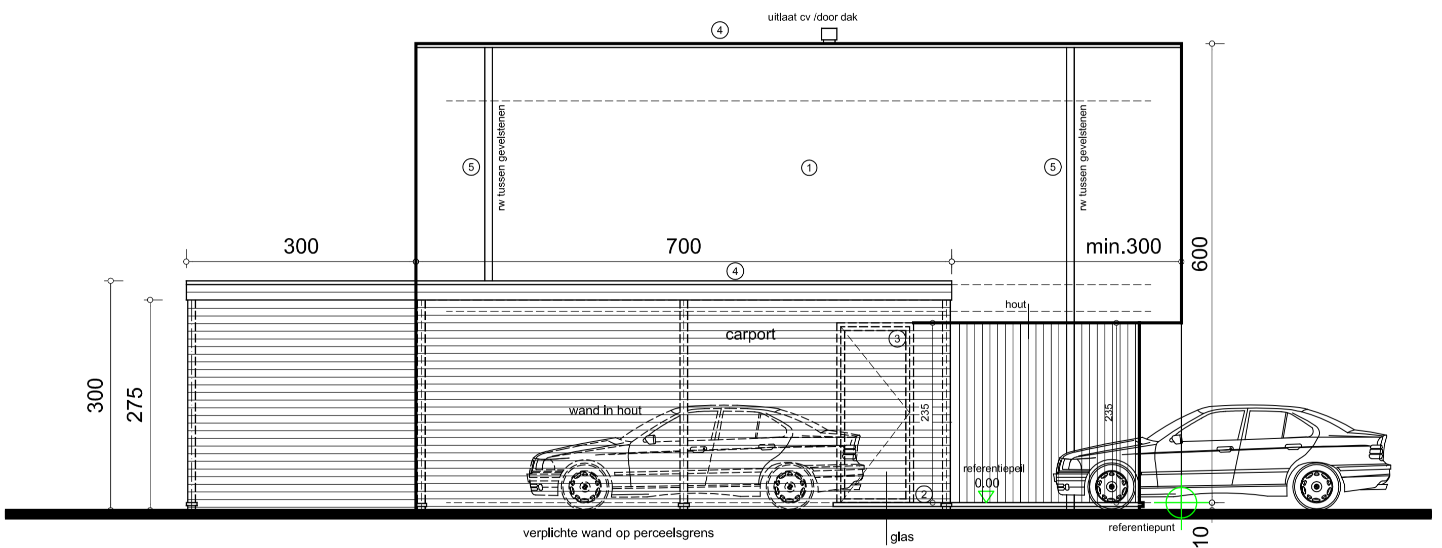
zijgevel links / 1:50
